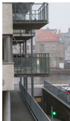
Viser innfesting mot sveiseplate mot fasade.
